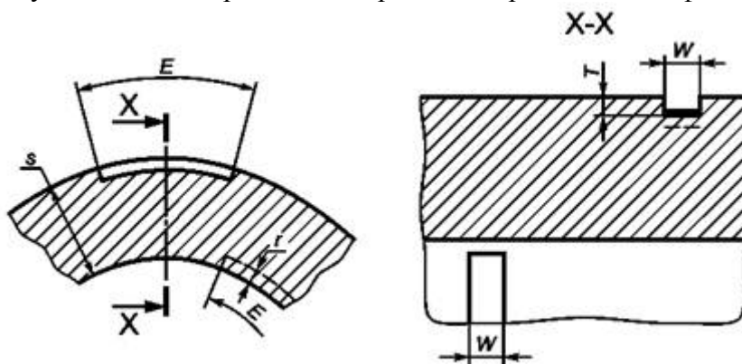
Рисунок В.1 - Контрольные надрезы для продольных дефектов
