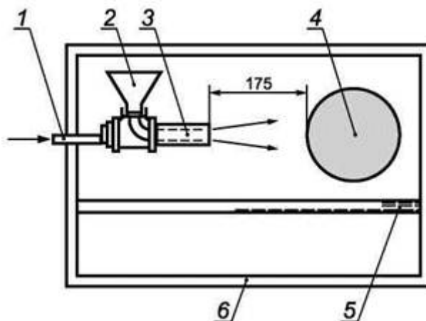
Рисунок F.1 - Установка для ударных испытаний гравием
